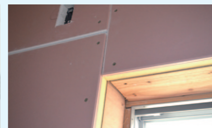
下地材への断熱複合パネル施工例
